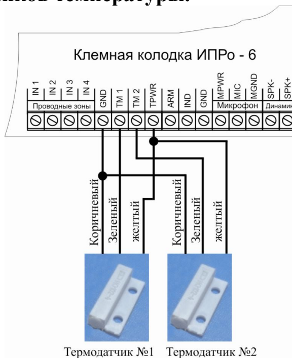
Подключения 2-х датчиков
