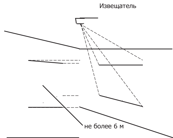
Рисунок 7 - Установка извещателя на потолке (для блокировки оконных проемов в соседних стенах)
