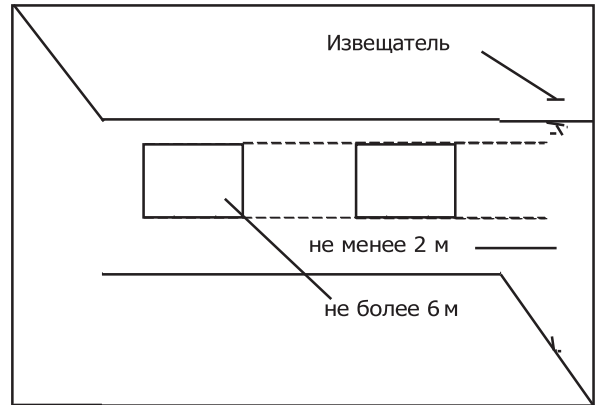
Рисунок 5 - Установка извещателя на боковой стене
