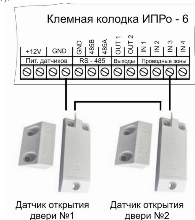
Подключение 2-х датчиков
