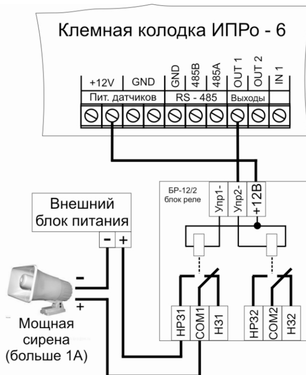
Подключение сирены с током потребления более 1А
