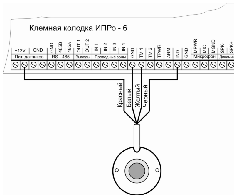
Считыватель ТМ
